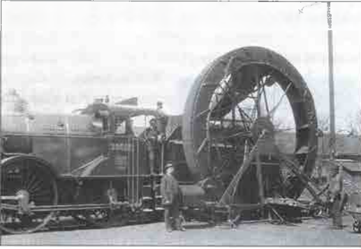
A Schilhan-féle szénemelő kerék, előtérben maga a feltaláló (T. Gy. M.)
